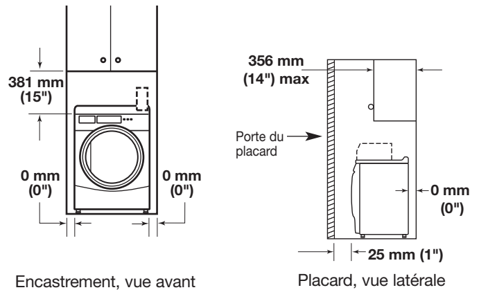
Encastrement, vue avant
