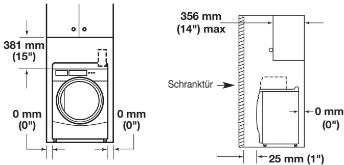
Vorderansicht Nischeneinbau
