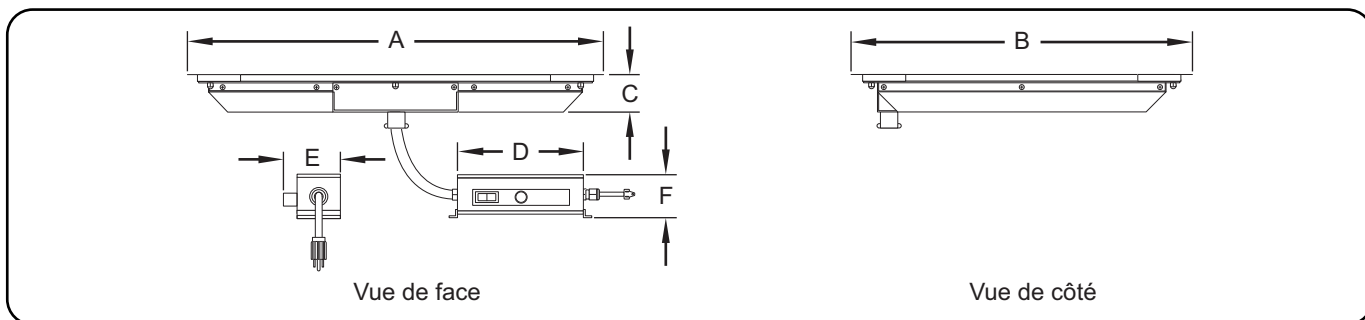
GRSSB Dimensions
